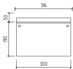
TYŁ
